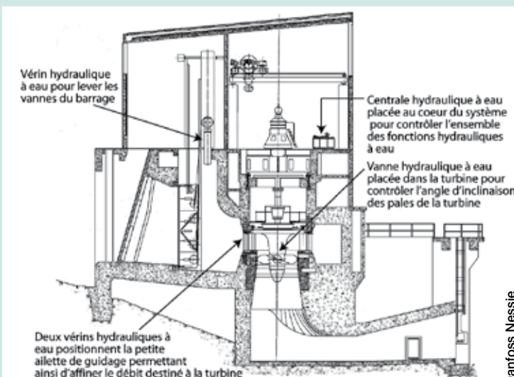
Une pompe hydraulique à eau est installée au cœur de la centrale hydroélectrique; les vérins et la régulation sont placés dans les différentes zones de travail.
